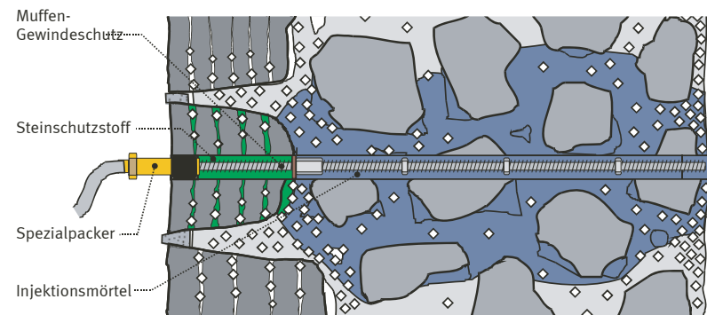
Einbringen des Steinschutzstoffes und Injektion eines ausgewählten Injektionsstoffes
